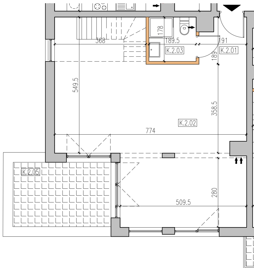
PIĘTRO 2
