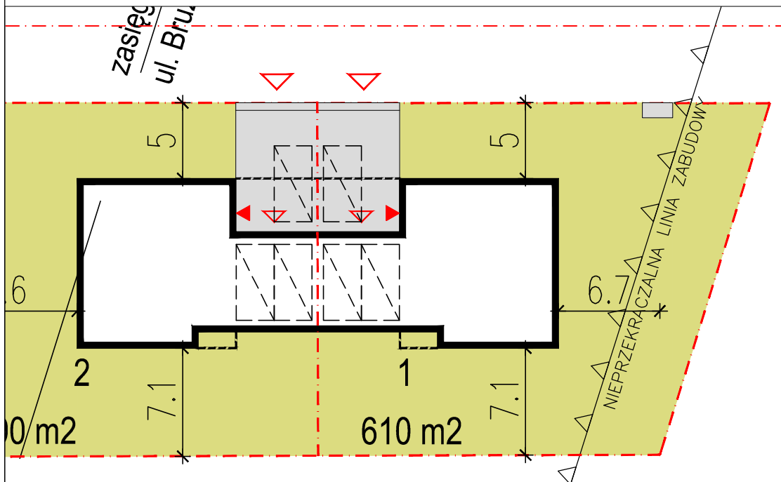
DZIAŁKA 1:1350
