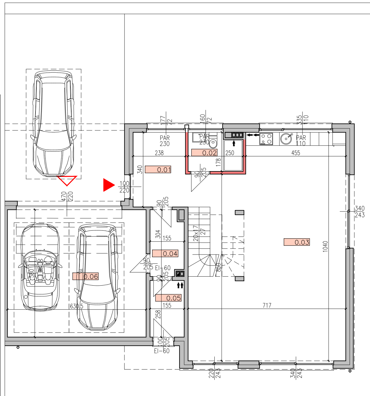
RZUT PARTERU 1:100
