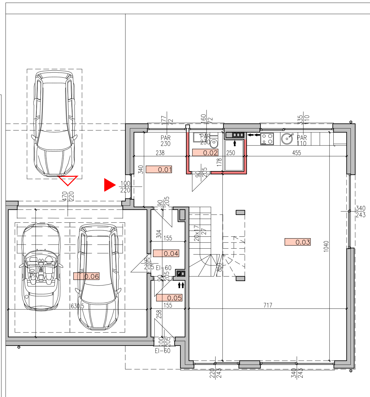
RZUT PARTERU 1:100
